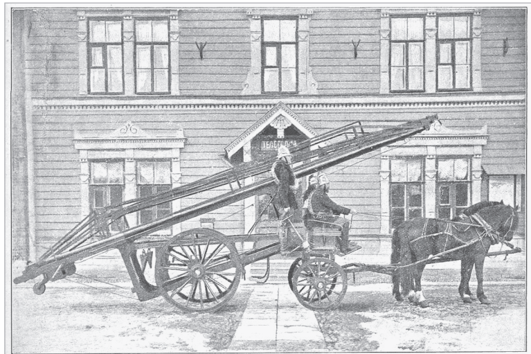
Рис. 205. Французская пожарная лестница в собранном виде.
